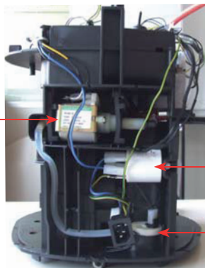
Płytki zasilacza
